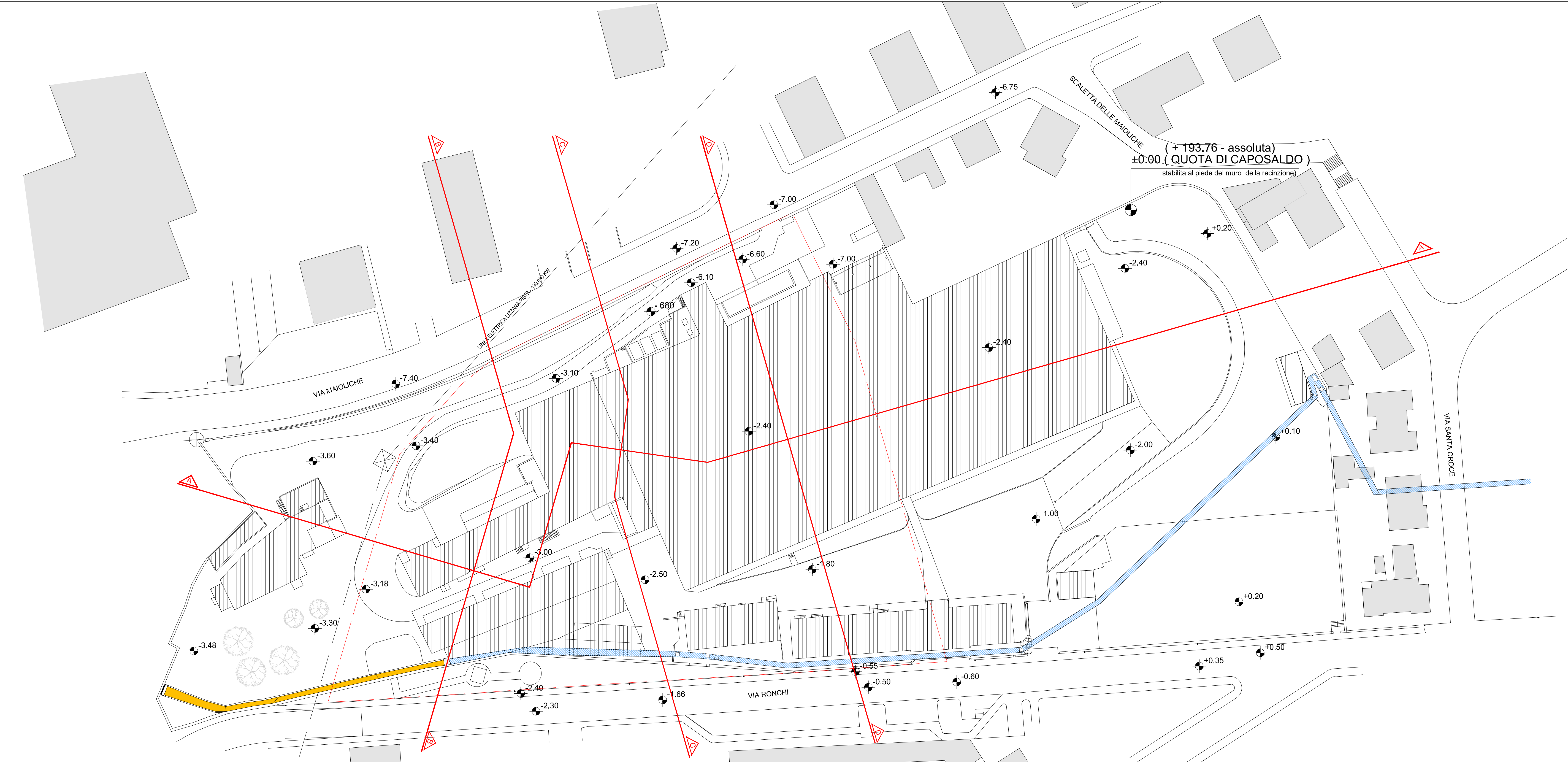
PLANIMETRIA DI RILIEVO
