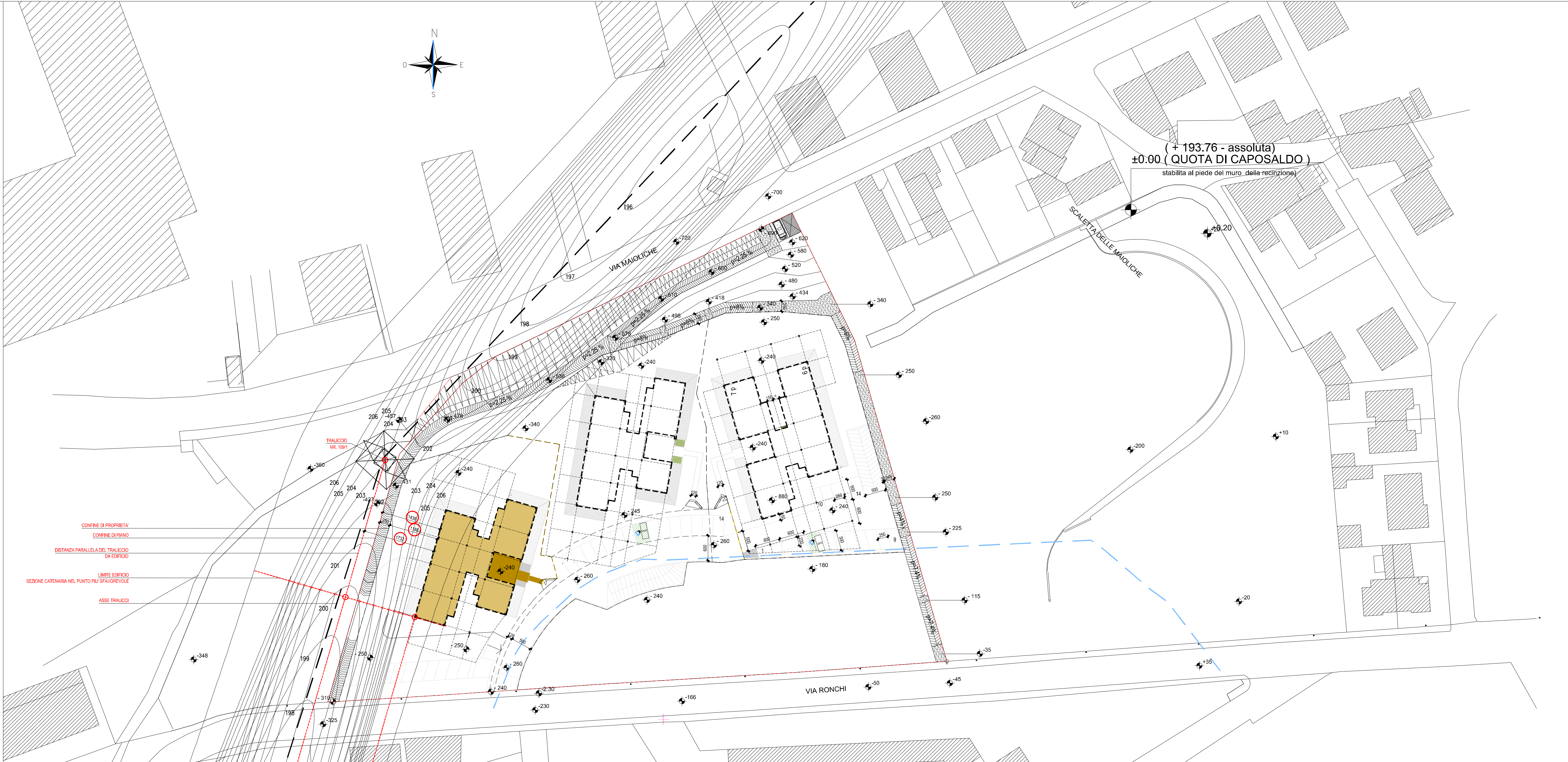
PLANIMETRIA DI PROGETTO - CON SOVRAPPOSIZIONE ISOLINEE a 3 mTESLA - Elettrodotto 132kV “Lizzana-Pista” Cod. 23100 - TERNA - PD
