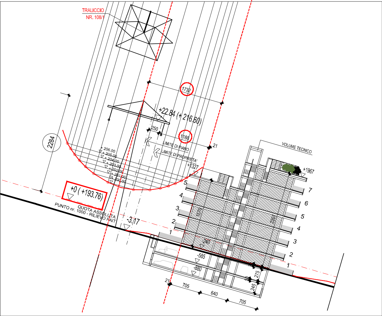
SEZIONE A-A - LINEA ELETTRICA CON ISOLINEA - 3 mTESLA
