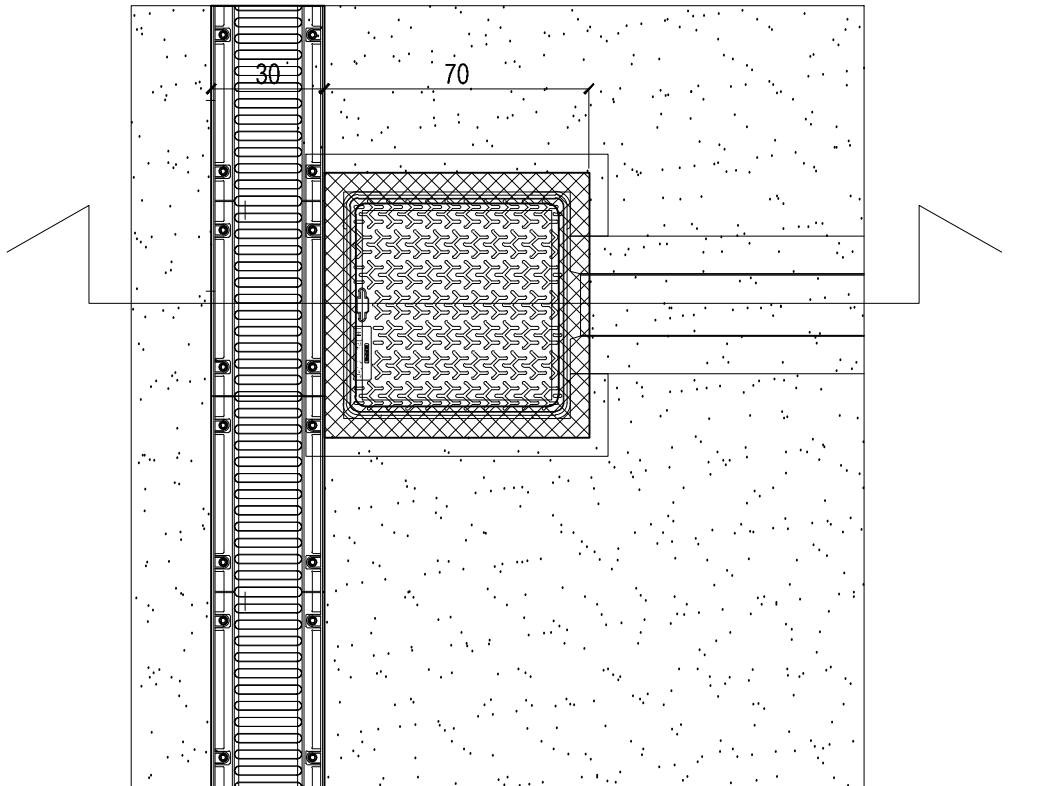
PIANTA
