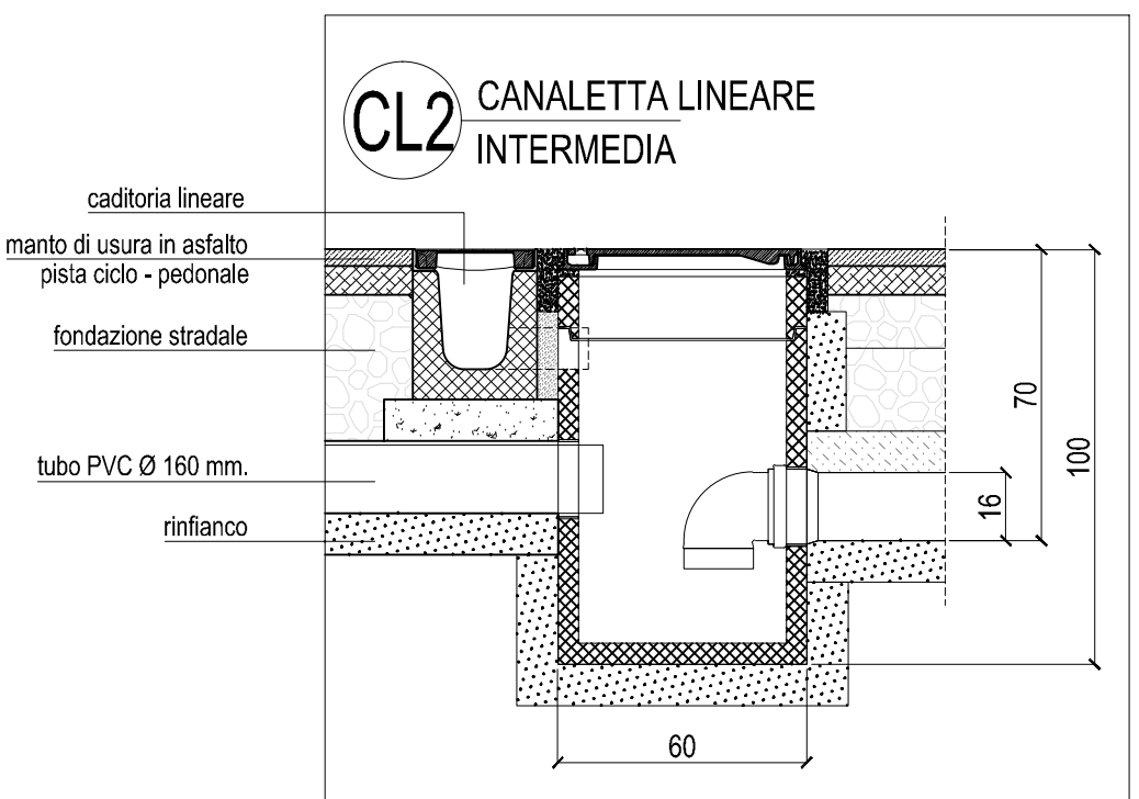
SEZIONE VERTICALE
