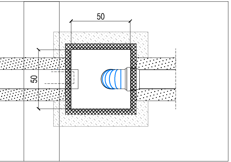
SEZIONE ORIZZONTALE
