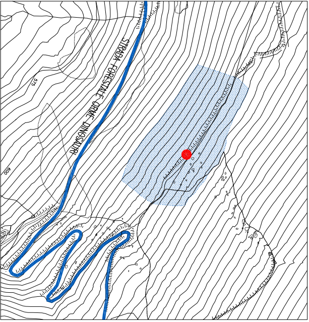
PLANIMETRIA CON INDIVIDUAZIONE DEL SITO – SCALA 1/5000
