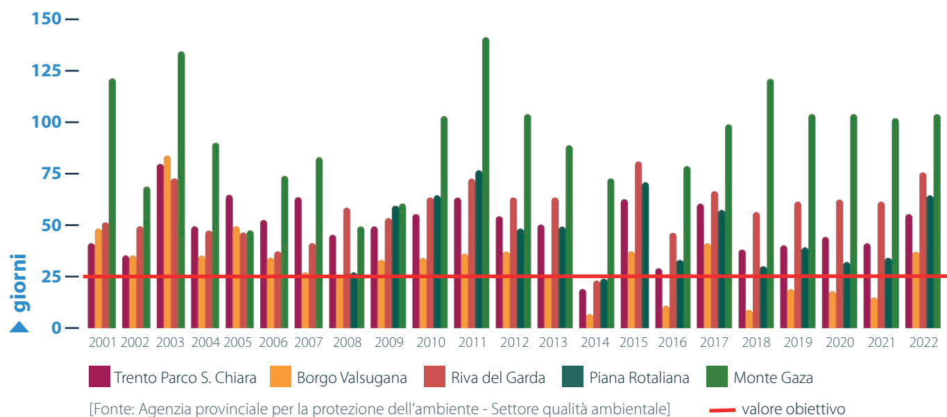
Figura 5.15: O 3 – superamenti del valore obiettivo
