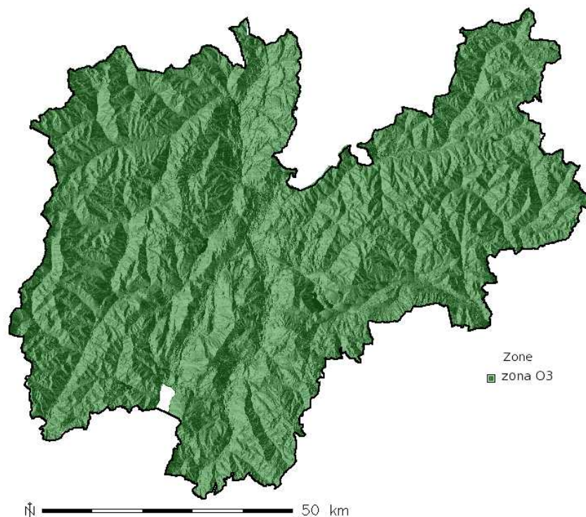
Fig. 3.2: Zonizzazione per la tutela della salute umana – O 3 .
