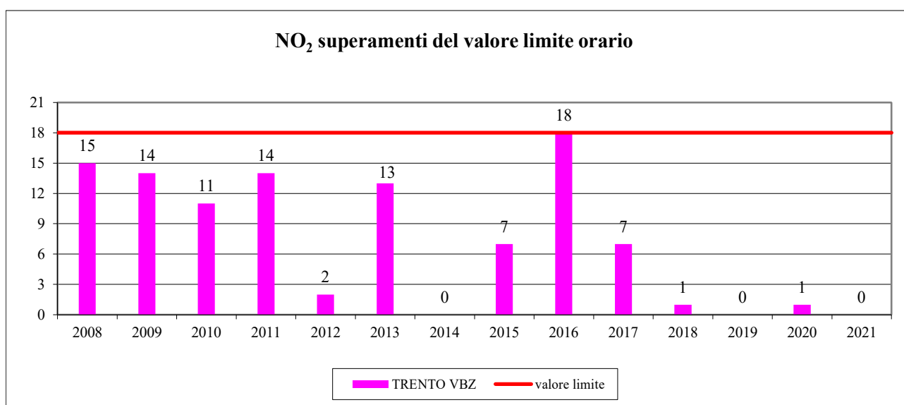
Fig. 5.1: \text{NO}_2 – superamenti del valore limite orario.
