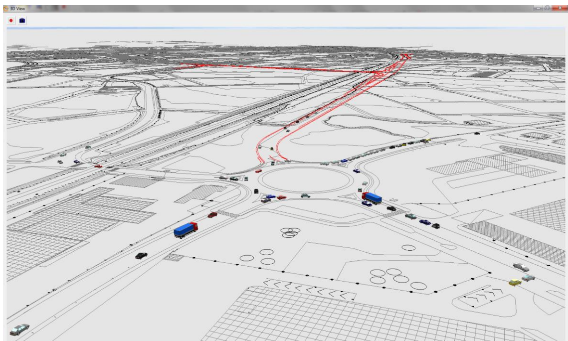
Figura 4.20 Microsimulazione Orvea Ingrosso – Screenshot dei video 2D e 3D delle simulazioni – SCENARIO 2.3
