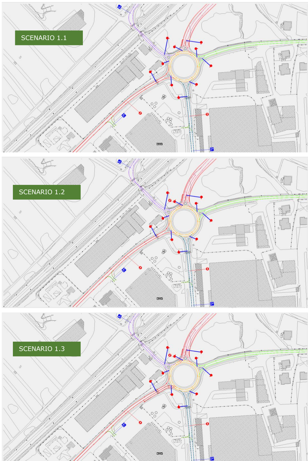
Figura 4.15 Microsimulazione Orvea Ingrosso – Scenari di progetto per Soluzione A
