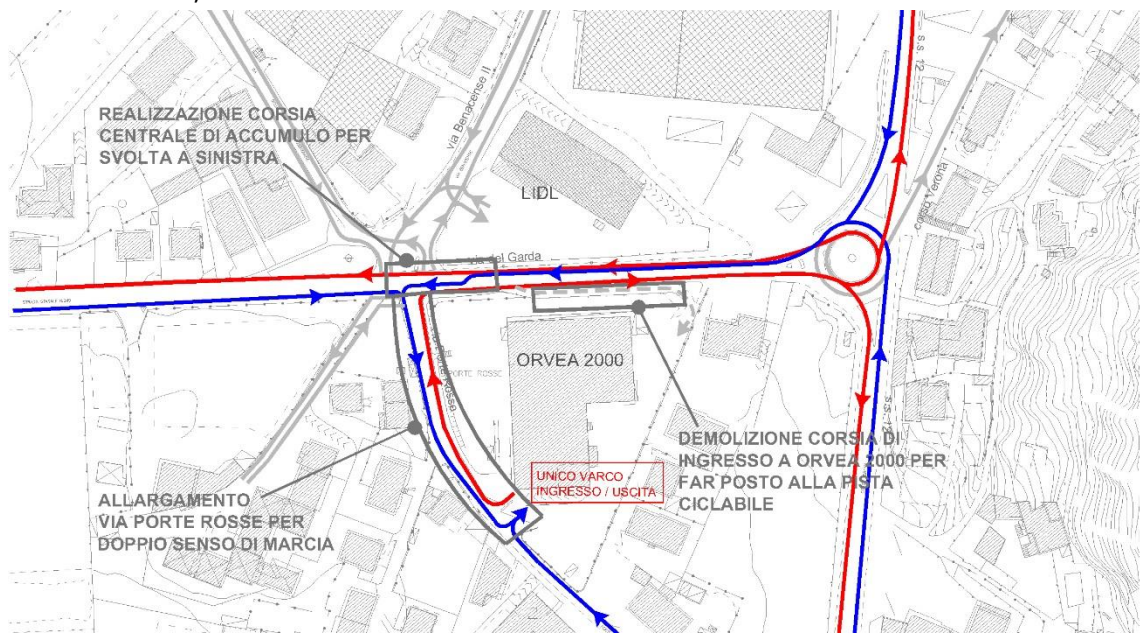
Figura 4.1 – Orvea 2000, accessi e recessi dalla struttura nello scenario di progetto, SOLUZIONE A.
