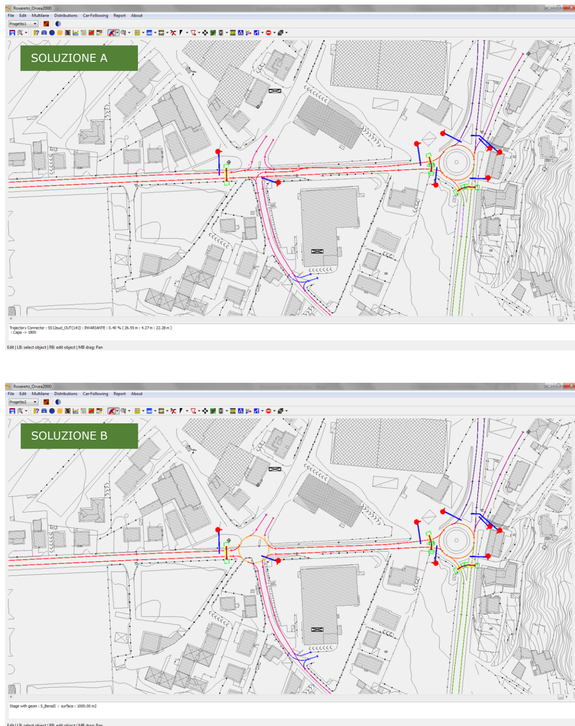
Figura 4.11 Microsimulazione Orvea 2000 – Rete di base per Stato Attuale e scenari di progetto
