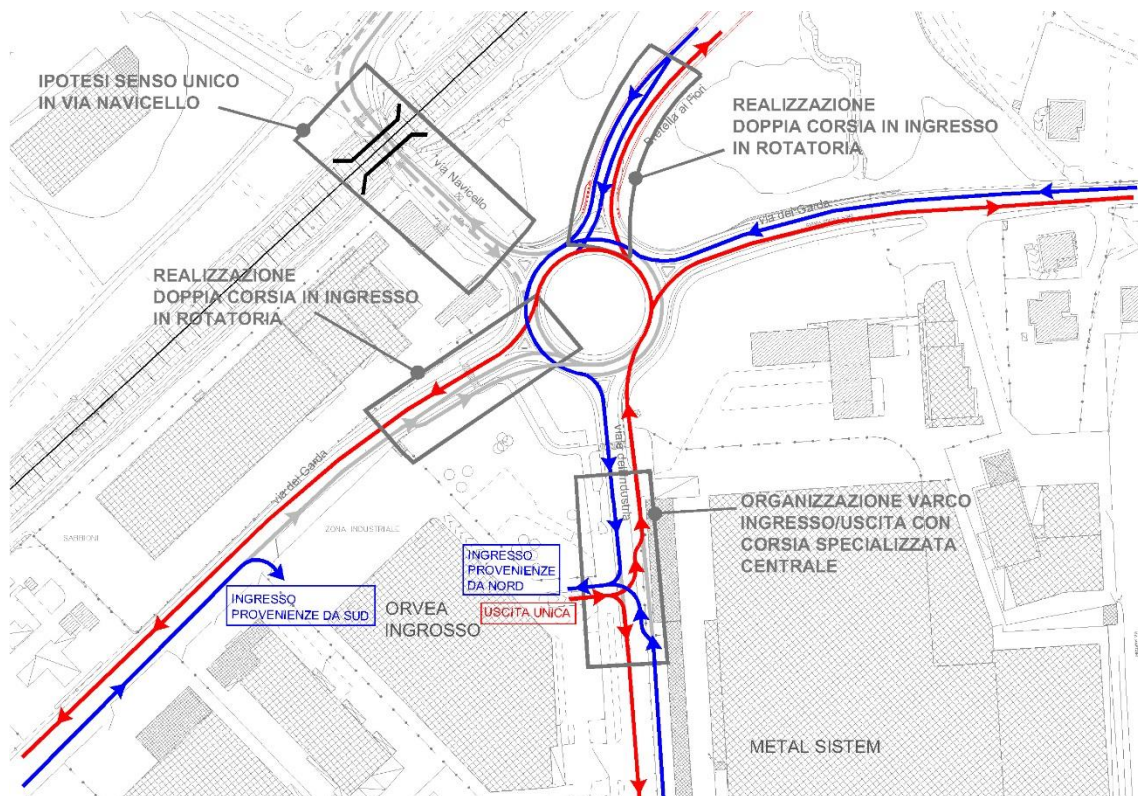
Figura 4.4 – Orvea Ingrosso, accessi e recessi dalla struttura nello scenario di progetto, SOLUZIONE B.
