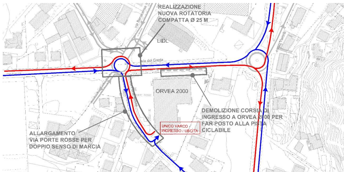
Figura 4.2 – Orvea 2000, accessi e recessi dalla struttura nello scenario di progetto, SOLUZIONE B.
