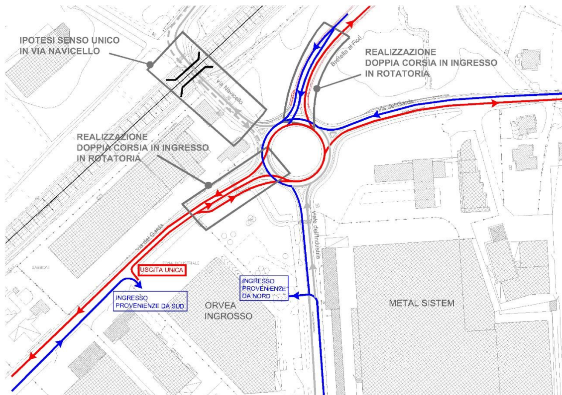
Figura 4.3 – Orvea Ingrosso, accessi e recessi dalla struttura nello scenario di progetto, SOLUZIONE A.
