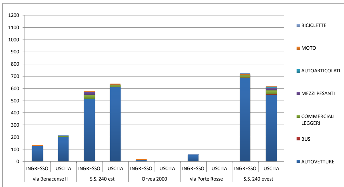
Figura 3.8 - Intersezione S.S.240 – via Benacense II – via Porte Rosse. Composizione del traffico veicolare privato sui diversi rami – ORA 17.30 –18.30
