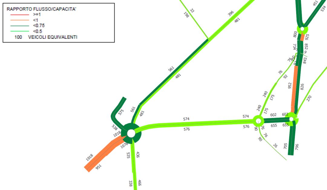
Figura 4.10 - Modello di simulazione del traffico - Differenze tra SCENARIO 3 e scenario BRETELLA AI FIORI.
