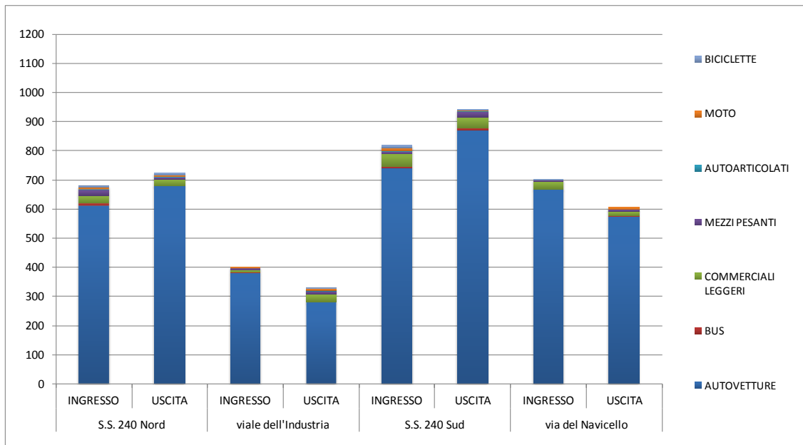
Figura 3.4 - Intersezione S.S.240 - S.S.12 - corso Verona. Composizione del traffico veicolare privato sui diversi rami - ORA 17.30 -18.30
