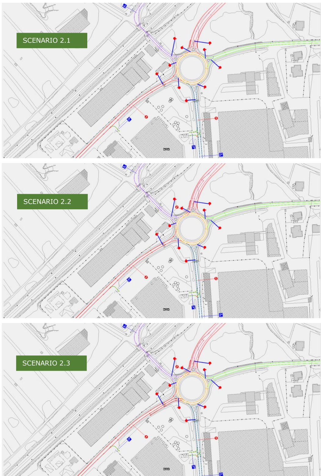
Figura 4.16 Microsimulazione Orvea Ingrosso – Scenari di progetto per Soluzione B
