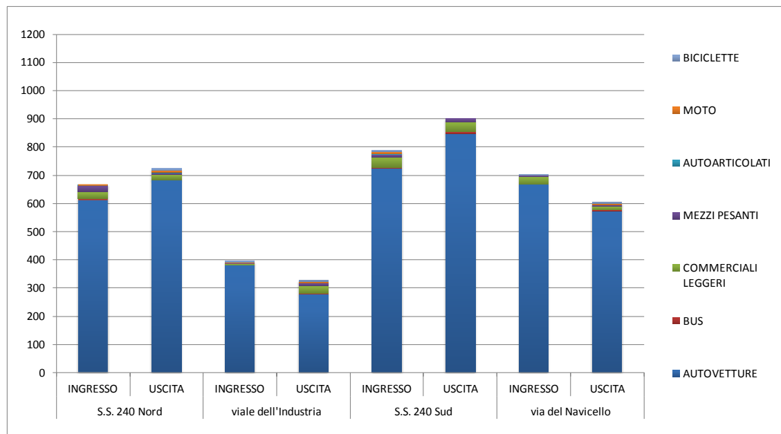
Figura 3.6 - Intersezione S.S.240 – via dell'Industria – via Navicello. Composizione del traffico veicolare privato sui diversi rami – ORA 17.30 –18.30
