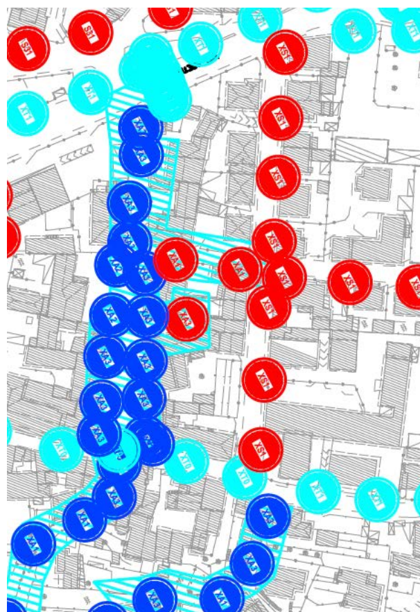
Figura 5: zone illuminotecniche omogenee - dettaglio
