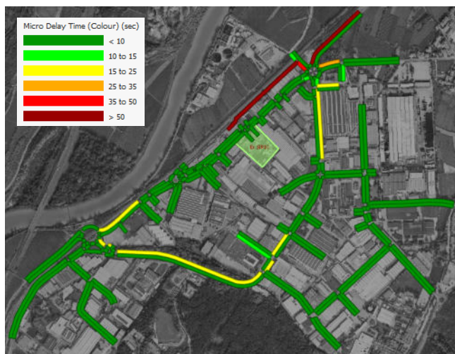
Figura 29 – Scenario di Progetto 01- Perditempo medio (17:00-18:00)
