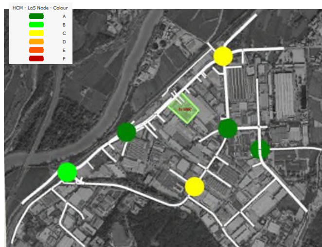
Figura 38 – Scenario di Progetto 02– Livelli di Servizio dei nodi (17:00-18:00)
