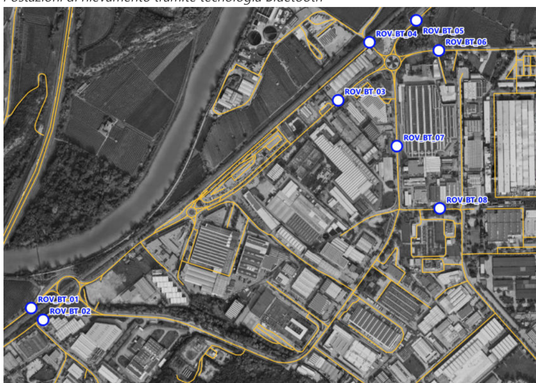
Figura 4 – Postazioni di rilevamento tramite tecnologia Bluetooth
