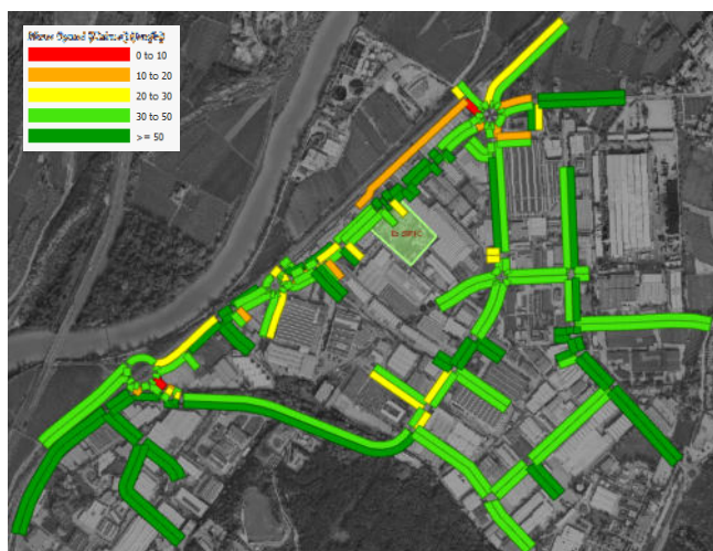
Figura 36 – Scenario di Progetto 02- Velocità media (17:00-18:00)
