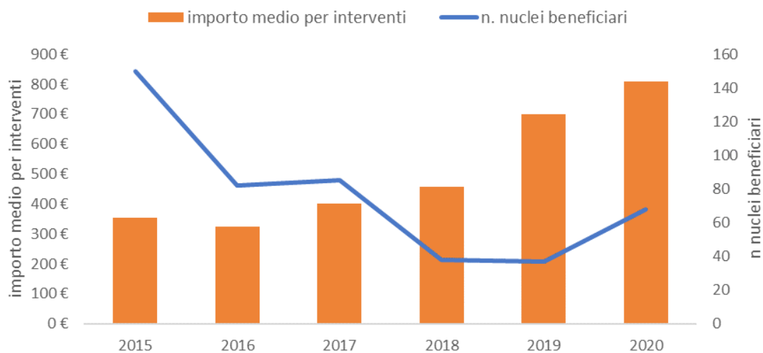
Figura 4. Importo medio degli interventi economici straordinari erogati dall'Ufficio servizi socio-assistenziali, area minori, e numero totale di beneficiari, anni 2015-2020
