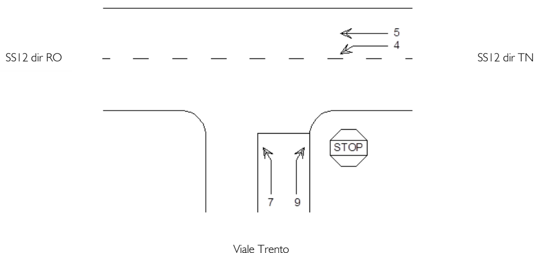
Schema delle manovre della intersezione e tre bracci
