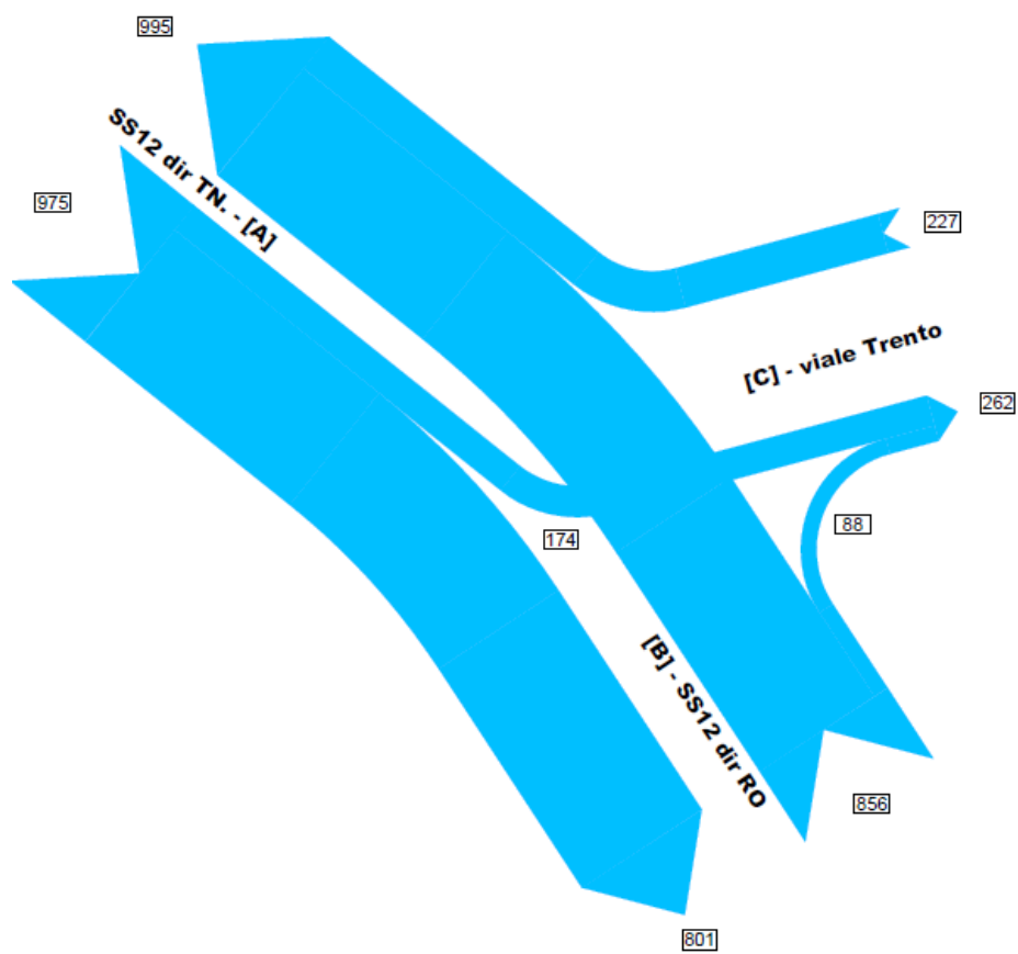
fig. 4 Flussogramma incrocio 02 a T esistente – stato attuale
