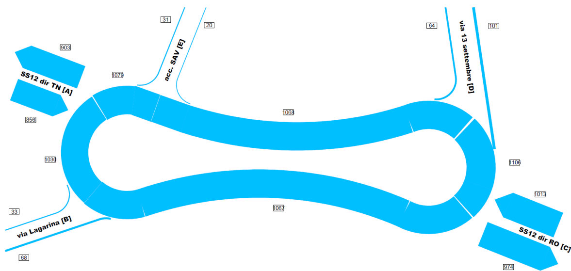
fig. 3 Flussogramma incrocio 01 in rotatoria – stato attuale
