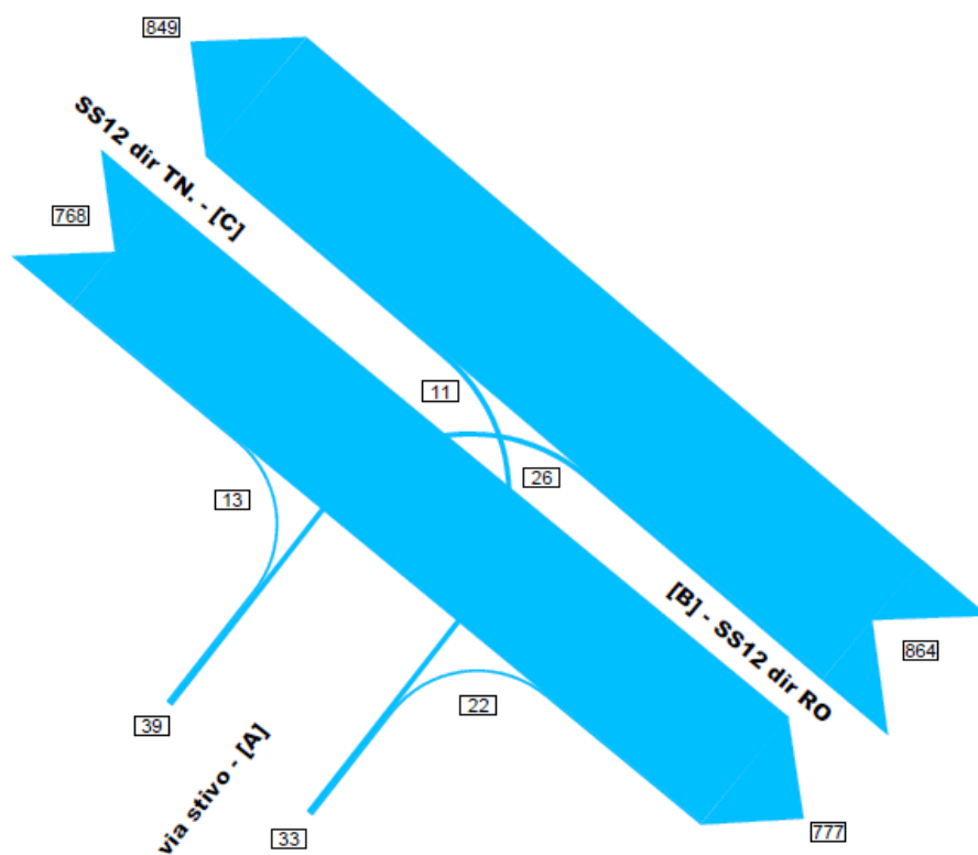
fig. 5 Flussogramma incrocio 03 a T esistente – stato attuale
