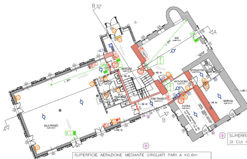
PIANTA PIANO TERRA Scala 1:100
