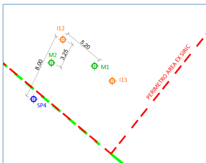
Figura 2.1: Planimetria campo prove
